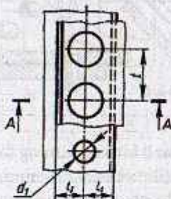
Bir qatorli ustma-ust chok d=\delta+8\text{MM} ; d_1=1,1d ; t=2\delta+8\text{MM} L_1=1,5\delta ; L=2\delta+1,5d (L-o'rnatilmagan parchin mix uzunligi)
