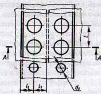
Ikki tomonlama taglikli uchma-uch chok d=\delta+8\text{MM} ; d_1=1,1d ; t=2\delta+8\text{MM} L_1=1,5d ; d_2=0,8d ; L=\delta+2d_2+1,5d (L-o'rnatilmagan parchin mix uzunligi)
