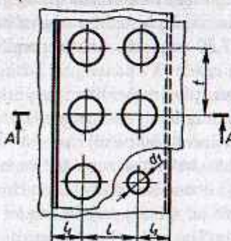
Ikki qatorli parallel ustma-ust chok d=\delta+8\text{MM} ; d_1=1,1d ; t=2,6\delta+15\text{MM} L=0,6t ; L_1=1,5d ; L_1=2\delta+1,5d (L-o'rnatilmagan parchin mix uzunligi)
