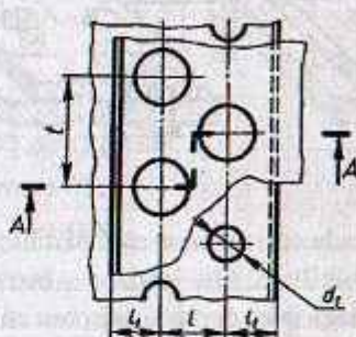
Shaxmat tartibidagi ustma-ust chok d=\delta+8\text{MM} ; d_1=1,1d ; t=2,6\delta+15\text{MM} L_1=1,5\delta ; L=0,6t ; L=2\delta+1,5d (L-o'rnatilmagan parchin mix uzunligi)
