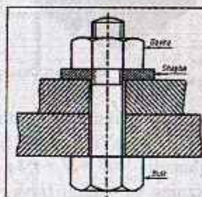
Shakl 17.18 - Gaykaning sekiyalı bosh ko'rinishi. Bolt va shaybaning qismli pozitsiyasi
