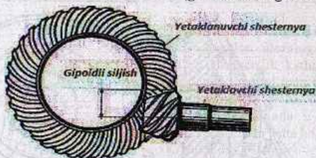
Gipoidli uzatmaning ustdan ko'rinishi
