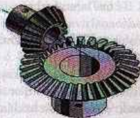
O'qlari o'zaro kesishgan konus tishli uzatma (g'ildiraklar to'g'ri tishli)
